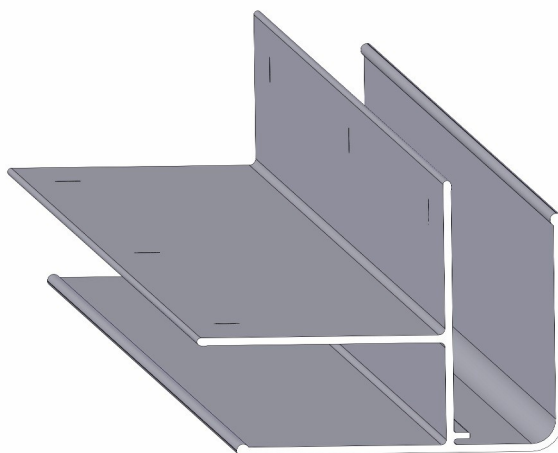
Corner Post (1x) fig B
